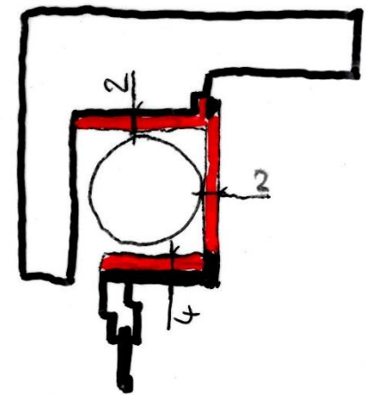
Abbildung 8: Dämmung im Bereich des längeren Rollladens: Seitlich und oben ist nur Platz für 2 cm Wärmedämmung.
