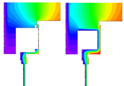
Abbildung 9: Wie viel die Dämmung bringt, kann mit einem Wärmestromprogramm berechnet werden. Die Abbildung zeigt das Ergebnis so einer Berechnung. Blau bedeutet dabei: hier ist es kalt (-10 °C), rot bedeutet warm (20 °C). Im rechten Bild mit der Dämmung bleibt es innen viel wärmer. Weniger Energie geht verloren.
