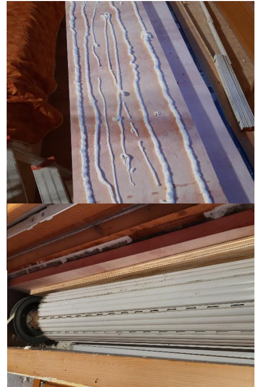
Abbildung 16: Platte positionieren und einkeilen.
