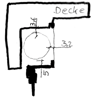
Abbildung 4: Die Zeichnung: Oben: die Ansicht von vorne ohne den Deckel. Unten: Schnitte durch den Kasten (links ist außen, rechts ist innen). In diesen Schnittzeichnungen ist unten das Fenster zu sehen, oben die Decke. Alle Maße in Zentimeter.
