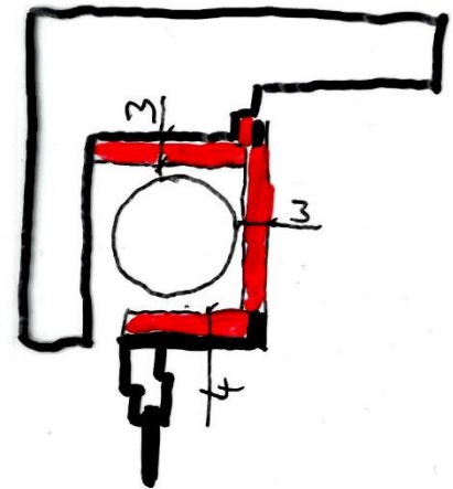
Abbildung 7: Dämmung (rot) im Bereich des kürzeren Rollladens.
