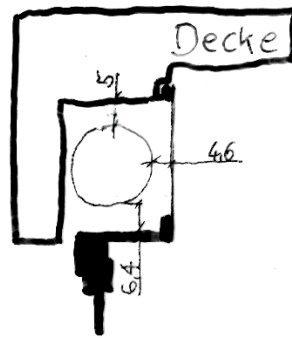
Abbildung 4: Die Zeichnung: Oben: die Ansicht von vorne ohne den Deckel. Unten: Schnitte durch den Kasten (links ist außen, rechts ist innen). In diesen Schnittzeichnungen ist unten das Fenster zu sehen, oben die Decke. Alle Maße in Zentimeter.
