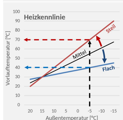
Abbildung 3: Steilheit der Heizkennlinie
